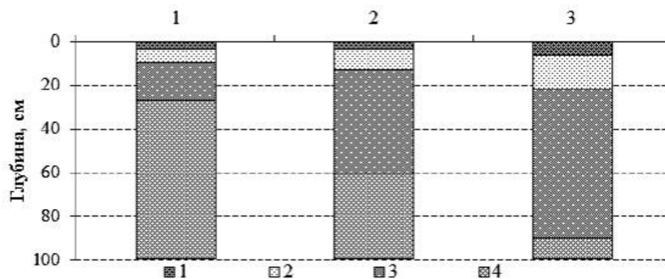
Рис. 2. Схема строения почвенных профилей: 1 – грубогумусовый, 2 – подзолистый, 3 – иллювиально-железистый горизонт, 4 – материнская порода
