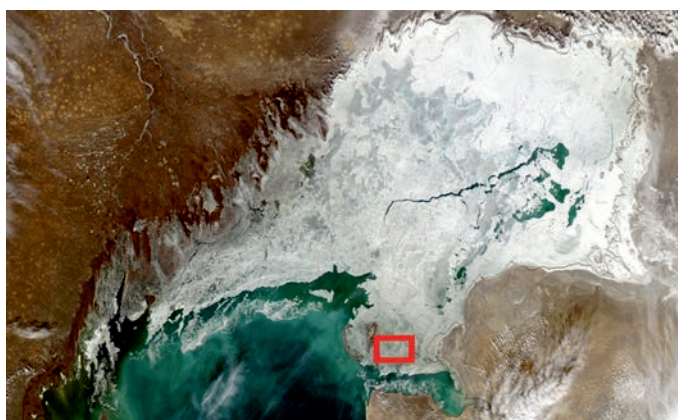
Рис. 2. Каспийское море: вверху — борозды ледового выпаживания на фрагменте снимка Landsat 8 [20], размер фрагмента 10 \times 16 км; внизу — местоположение фрагмента (район Тюленьих островов) на обзорном снимке Северного Каспия ИСЗ AQUA от 5.02.2015 г.
