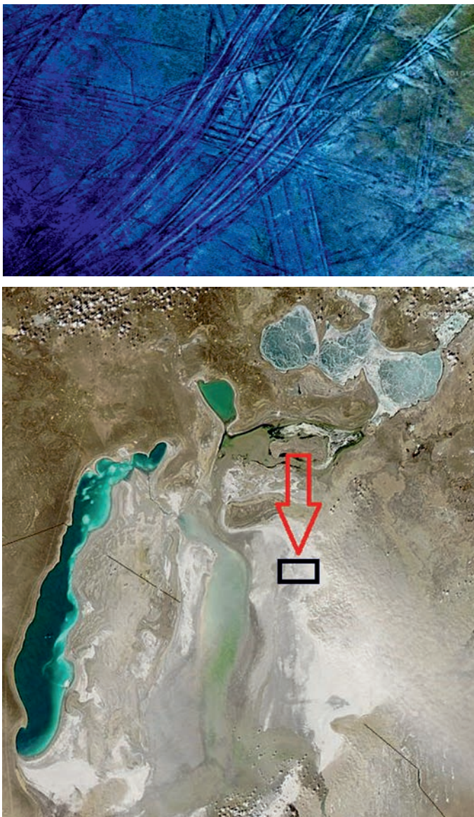
Рис. 3. Аральское море: вверху — борозды ледового выпахивания на космическом снимке современного побережья, размер фрагмента 1.5 \times 3 км [22]; внизу — местоположение фрагмента на обзорном космическом снимке 2010 г.
