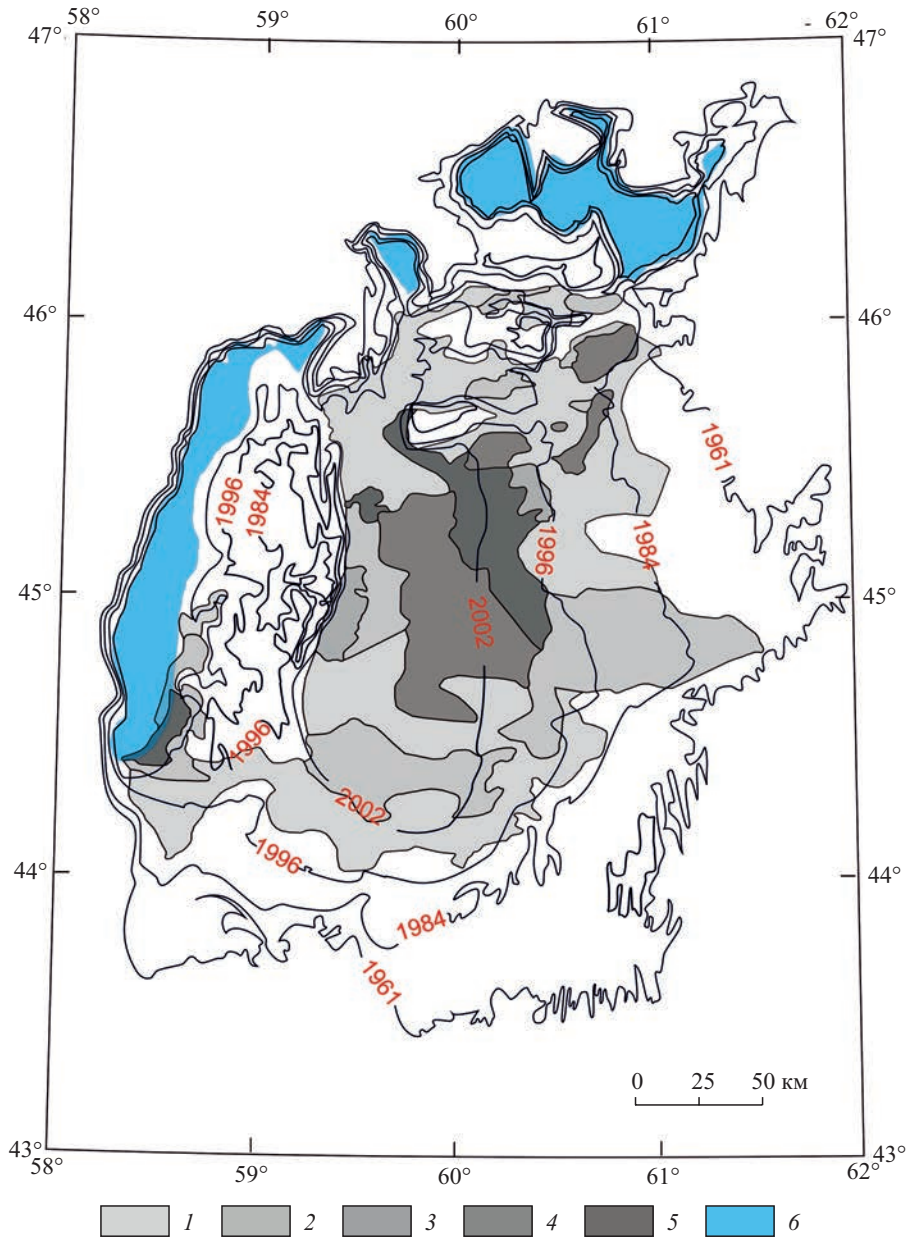
Рис. 6. Схема распространения ледово-эскарационного рельефа, наложенная на схему береговых линий (по [6]). Условные обозначения: 1 — покрытие дна бороздами менее 10 %, 2 — 10—20 %, 3 — 20—30 %, 4 — 30—50 %; 5 — более 50 %; 6 — современное положение Аральского моря.
