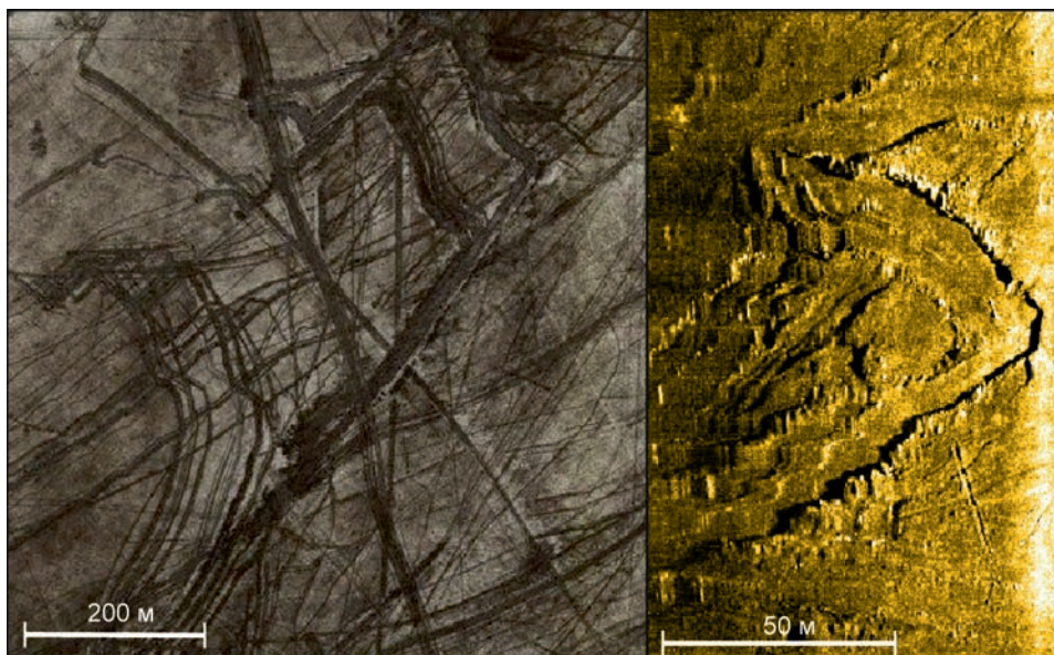
Рис. 10. Изгибающиеся ледово-эскарационные борозды на дне Аральского моря (спутниковый снимок WorldView-3, слева ) и Байдарацкой губы Карского моря (съемка ГБО, справа ).
