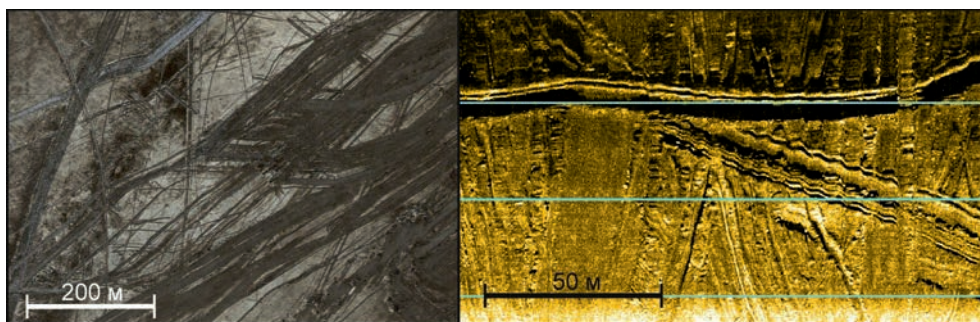
Рис. 11. Пересекающиеся ледово-эскарационные борозды на дне Аральского моря (спутниковый снимок WorldView-3, слева ) и Байдарацкой губы Карского моря (съемка ГБО, справа ).
