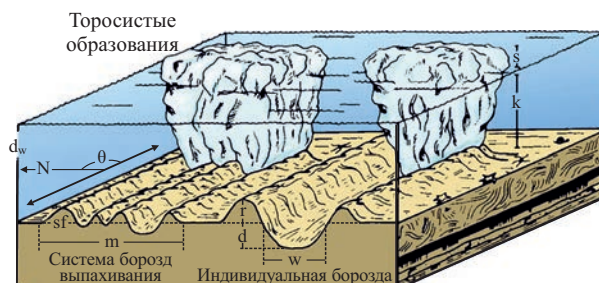
Рис. 1. Экзарация дна ледяными торсистыми образованиями [17]: k — глубина моря; s — высота торося; d — глубина борозды; w — ширина борозды; r — высота бортика обваловки; m — ширина системы борозд; sf — ширина бортика; \theta — ориентировка борозды.
