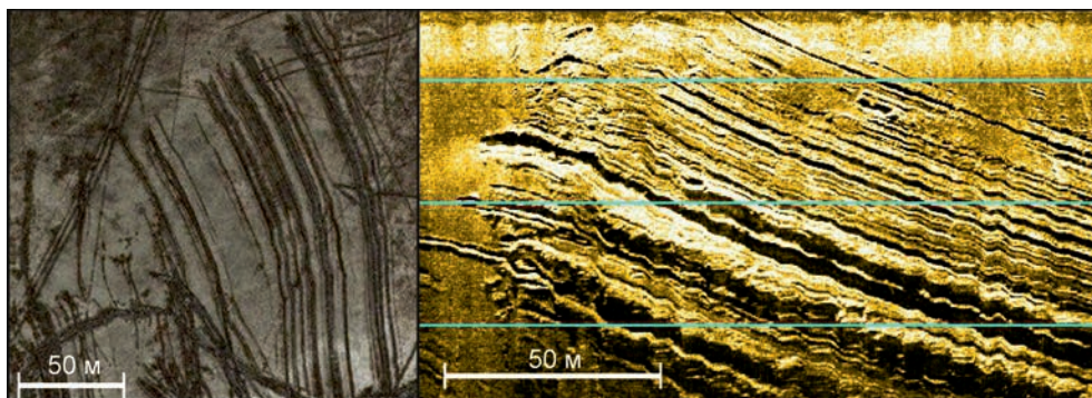
Рис. 8. «Гребенки» ледово-экзарационных борозд на дне Аральского моря (спутниковый снимок WorldView-3, слева ) и Байдарацкой губы Карского моря (съемка ГБО, справа ).
